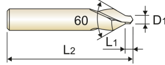
Form A (D1303, \emptyset 0.5 , \emptyset 0.8 )
